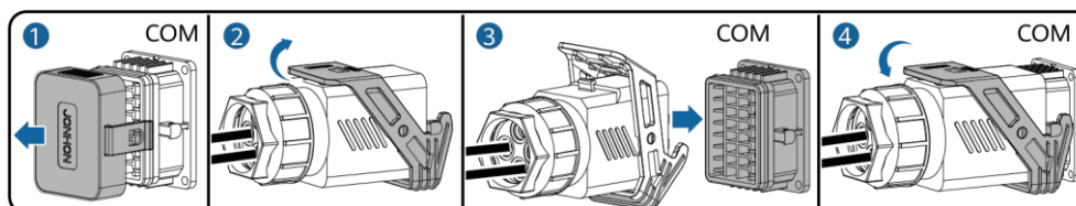
Kommunikationsport (COM)
