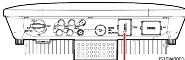
Kommunikationsport (COM)
