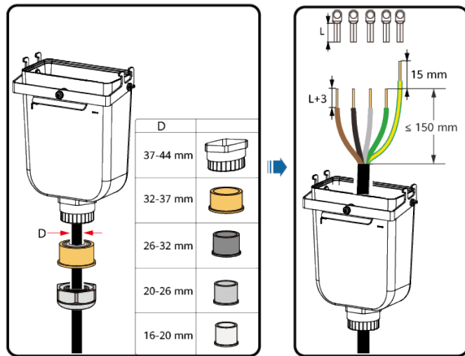
Abbildung 5-5 Abisolieren des Netzkabels (verwenden Sie beispielsweise ein fünfadriges Kabel)
