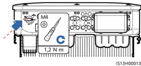
Abbildung 4-14 Montieren der Sicherungsschraube für den DC-Schalter
