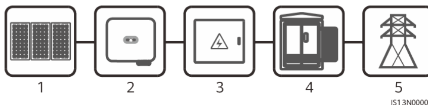
Abbildung 2-2 Netzwerkanwendung – Szenario mit einem einzelnen Wechselrichter
