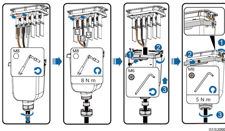
Abbildung 5-9 Dreidriges Kabel (L1, L2 und L3)
