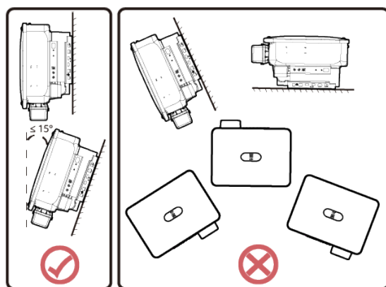
Abbildung 4-1 Montagewinkel
