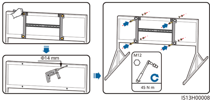
Abbildung 4-11 Sichern der Montagehalterung
