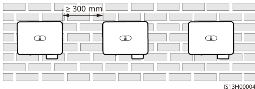
Abbildung 4-3 Horizontale Montage (empfohlen)
