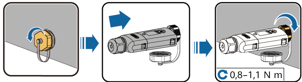
Abbildung 5-13 Anschließen eines WLAN-FE Smart Dongle (WLAN-Kommunikation)
