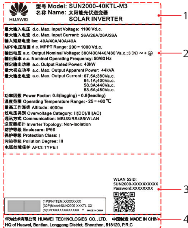
Abbildung 2-5 Typenschild
