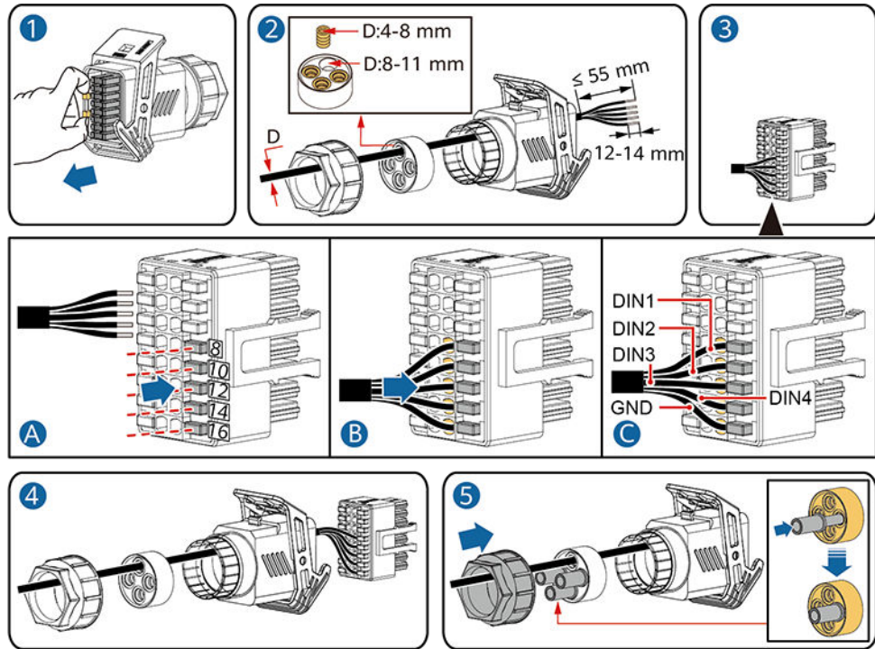
Abbildung 5-24 Anschließen des Kabels
