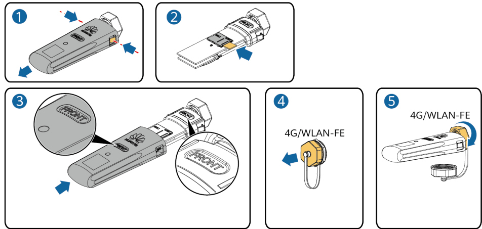
Abbildung 5-12 Anschließen eines 4G Smart Dongle
