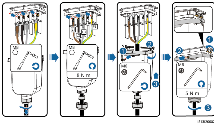
Abbildung 5-7 Vieradriges Kabel (L1, L2, L3 und PE)
