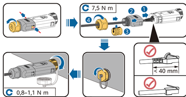
Abbildung 5-14 Anschließen eines WLAN-FE Smart Dongle (FE-Kommunikation)
