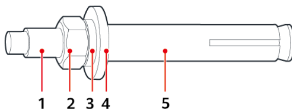
Abbildung 4-12 Aufbau einer Dehnschraube
