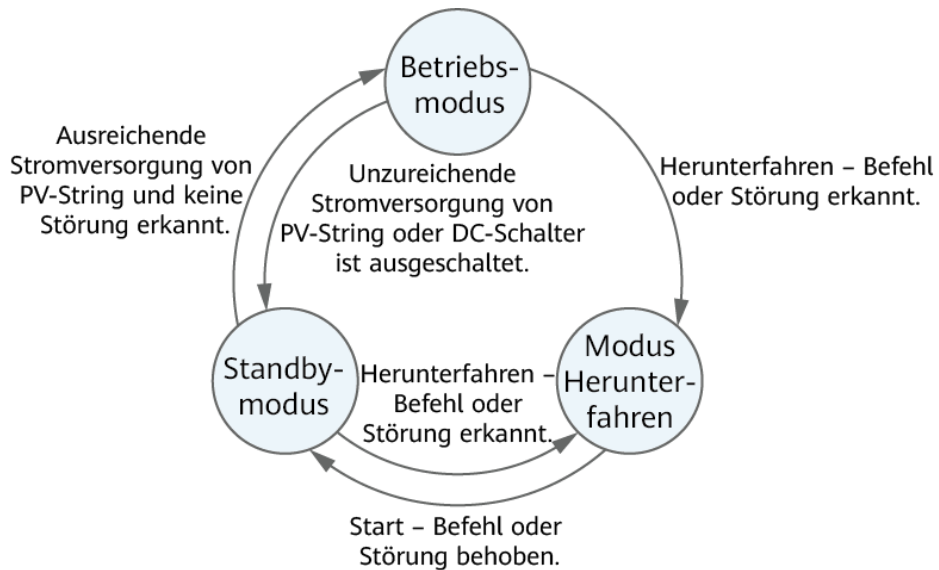
Abbildung 2-7 Arbeitsmodi
