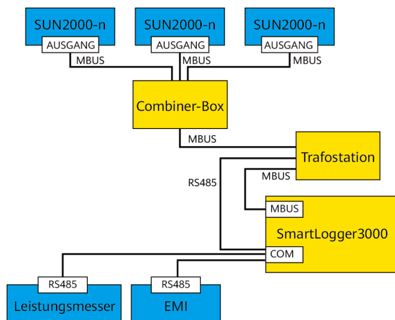
Abbildung 5-19 MBUS-Kommunikation
