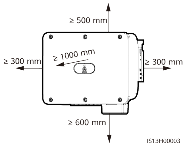
Abbildung 4-2 Montageabstände
