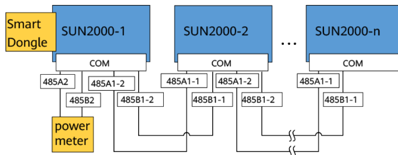
Abbildung 5-17 Smart Dongle-Netzwerkaufbau
